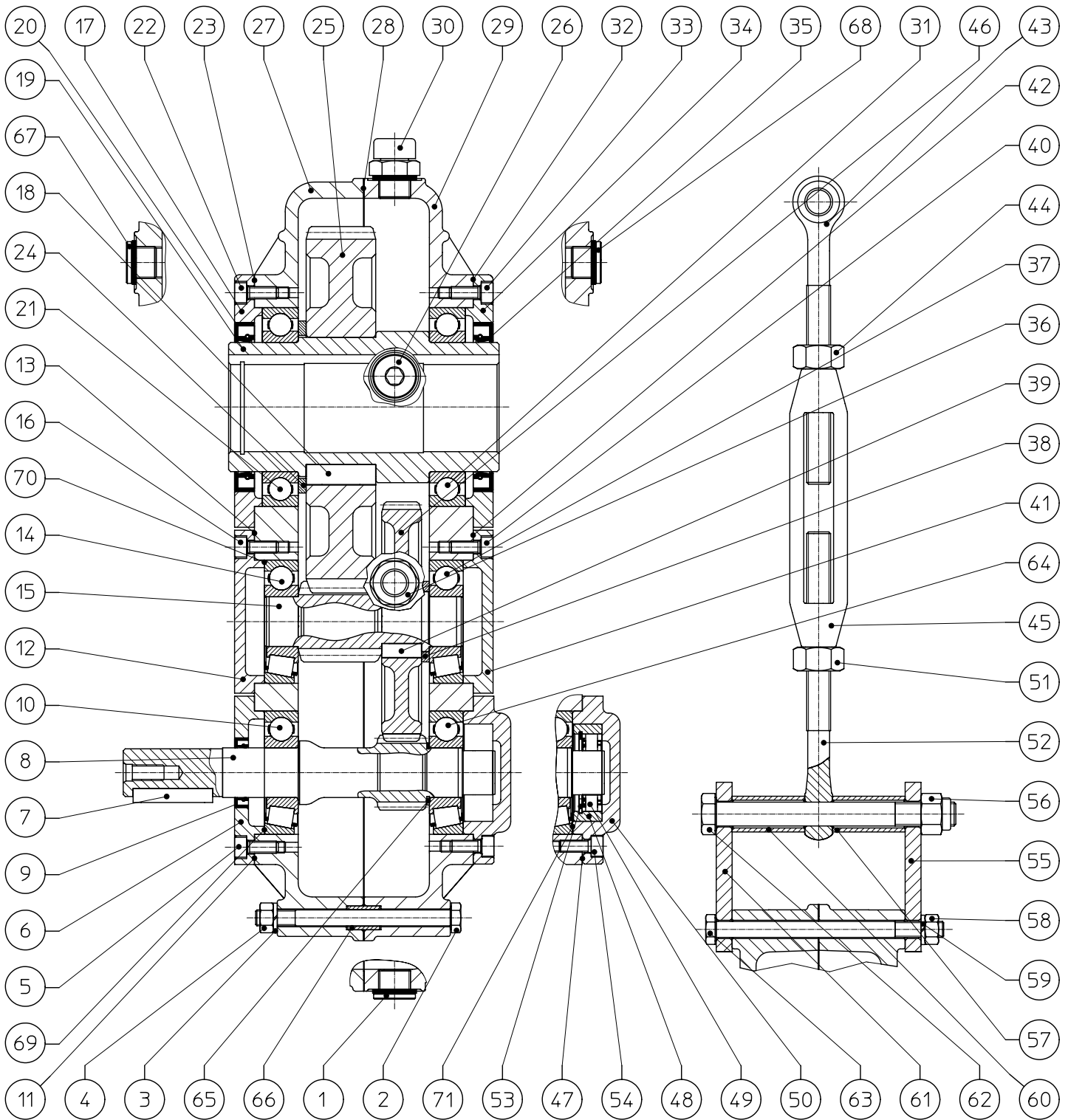
Particolari 67 e 68 a richiesta solo per riduttori in posizioni di lavoro VA e VB.
